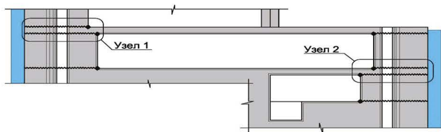
Рисунок 7.2.5 - Гидроизоляция швов бетонирования и швов сопряжения стен и перекрытий в машинном зале и технологических помещениях здания ГЭС (фрагмент 1 на рис. 6.1.1).
