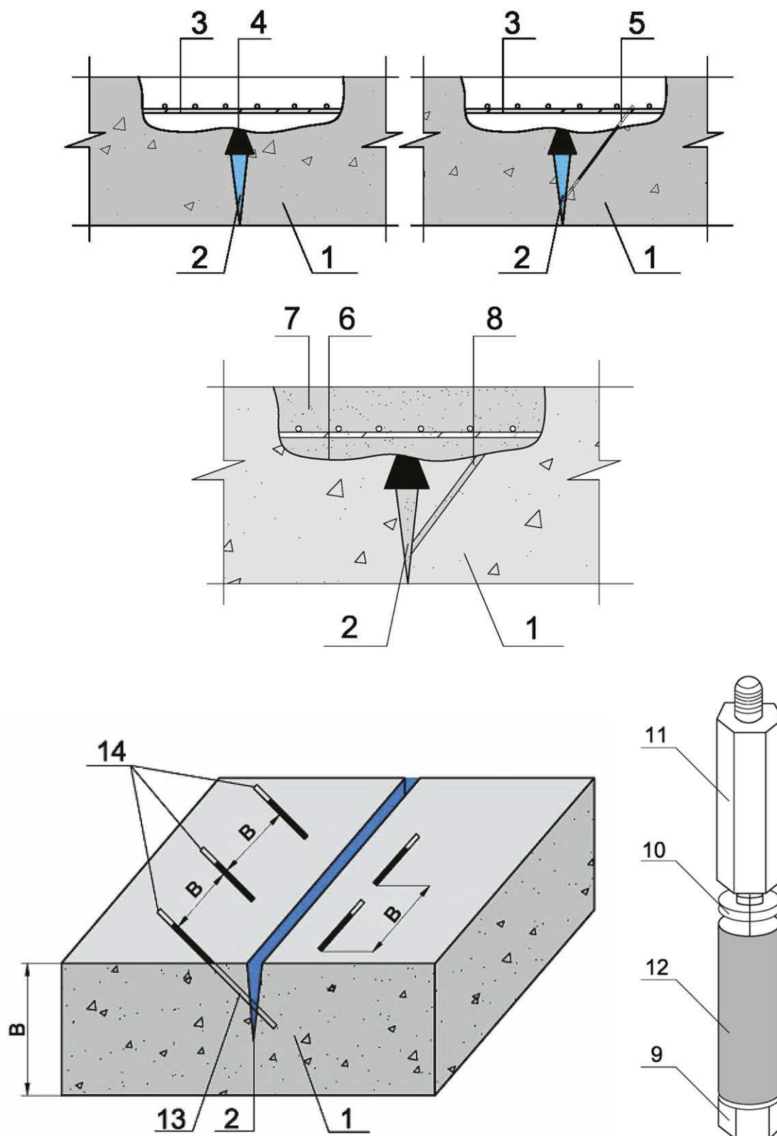
Рисунок 7.4.8 - Заполнение каверн, пустот и полостей в железобетонных конструкциях: 1 - железобетонная конструкция; 2 – водонесущая статическая трещина; 3 – арматура; 4 – гидропломба «Ватерплаг» («Пенеплаг»); 5 – инъектор; 6 – «Пенетрон»; 7 – «Скрепа М500 Ремонтная»; 8 – «Скрепа М600 Инъекционная»; 9 – болт с отверстием; 10 – прижимное кольцо (шайба); 11 – трубка инъектора; 12 – резиновый уплотнитель; 13 – шпур для установки инъектора; 14 – установка инъекторов в шахматном порядке.
