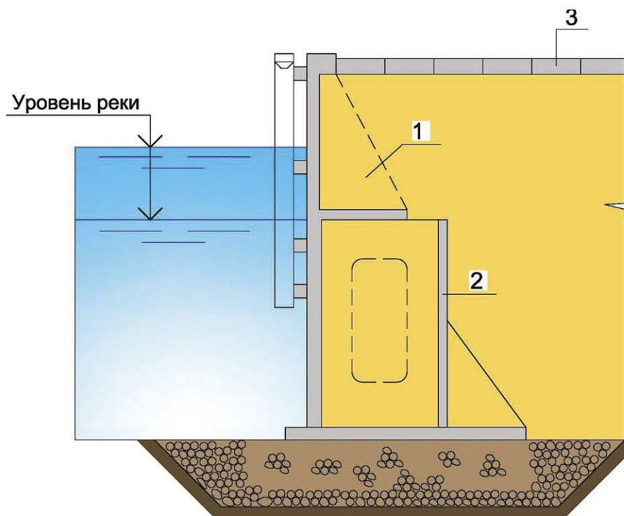
Рисунок 6.5.1 - Конструкция причального сооружения из железобетонных массивов-гигантов:
