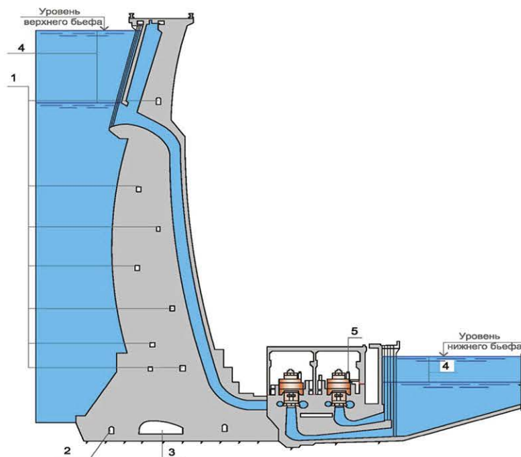
Рисунок 6.2.2 - Бетонная арочная плотина:
