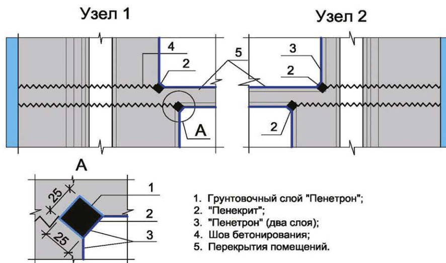
Рисунок 7.2.6 - Типовые узлы гидроизоляции в машинном зале и технологических помещениях здания ГЭС (узлы 1 и 2 на рис. 7.1).
