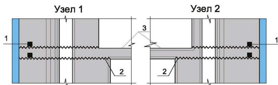
Рисунок 7.1.9 – Типовые узлы гидроизоляции в машинном зале технологических помещениях (узлы 1 и 2 на рис. 7.1.8):
