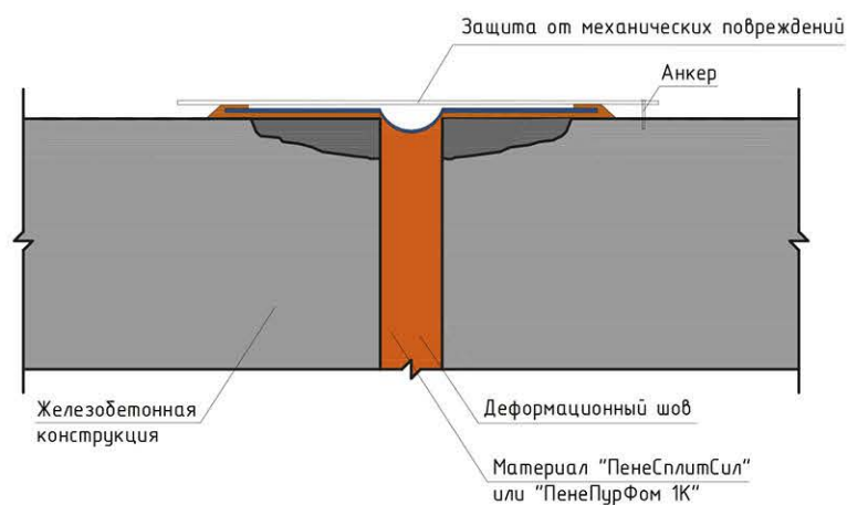
Рисунок 7.3.16 – Защита ленты от механических воздействий.
