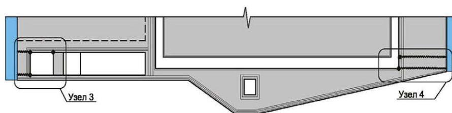
Рисунок 7.2.7 - Гидроизоляция швов бетонирования и швов сопряжения стен и перекрытий в потернах, смотровых шахтах и соединительных коридорах здания ГЭС (фрагмент 2 на рис. 6.1.1).
