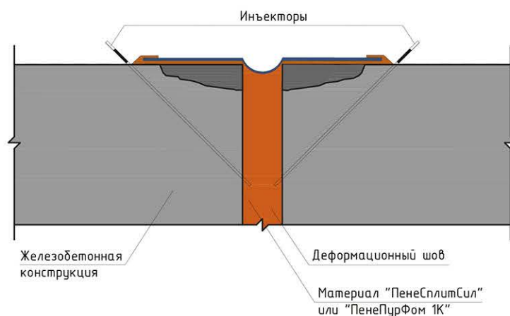
Рисунок 7.3.15 - Заполнение полости шва инъекционными смолами.
