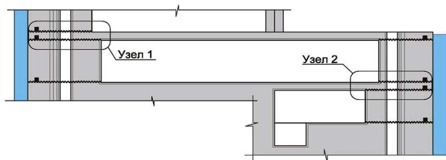
Рисунок 7.1.8 – Схема расположения швов бетонирования и гидроизоляционного жгута «Пенебар» в местах сопряжения стен и перекрытий в машинном зале и технологических помещениях здания ГЭС (фрагмент 1 на рис. 6.1.1).
