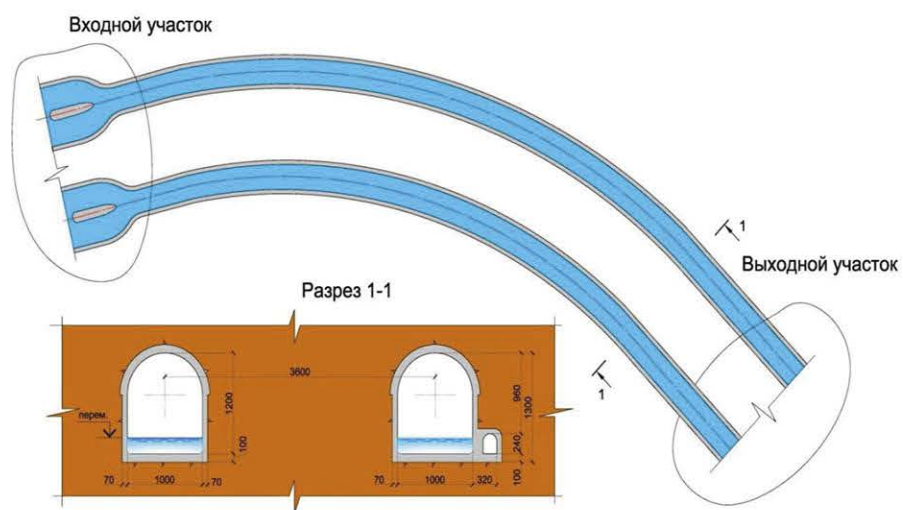
Рисунок 6.7.1 - Водосбросные туннели:
