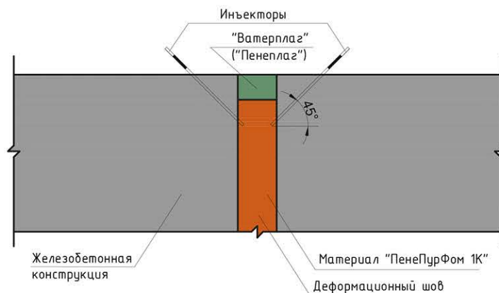
Рисунок 7.3.17 - Устранение течей через полость деформационного шва.
