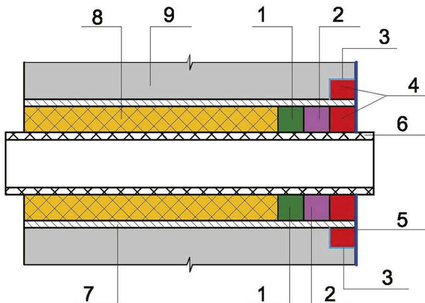
Рисунок 7.2.52а - Гидроизоляция места ввода коммуникаций:
