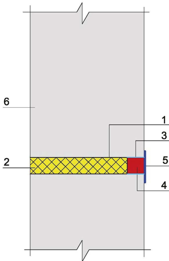
Рисунок 7.2.57- Гидроизоляция технологических отверстий от стяжек опалубки:
