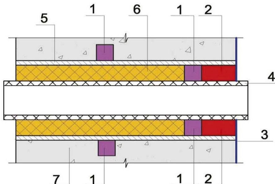
Рисунок 7.1.12 - Гидроизоляция места ввода коммуникаций: 1 - гидроизоляционный жгут «Пенебар»; 2 - «Пенекрит»; 3 - «Пенетрон»; 4 - коммуникационная труба; 5 - металлическая гильза; 6 - сальниковая набивка; 7 - железобетонная стена.
