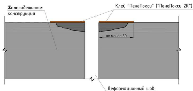
Рисунок 7.3.12 - Нанесение клея «ПенеПокси» («ПенеПокси 2К») на кромки деформационного шва.
