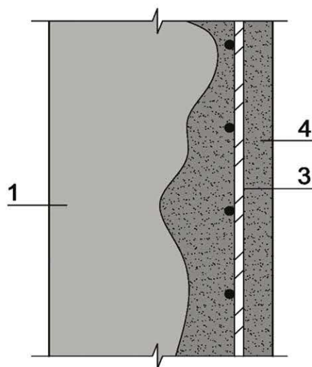
Рисунок 7.4.5 - Восстановление структурно поврежденного железобетона:
