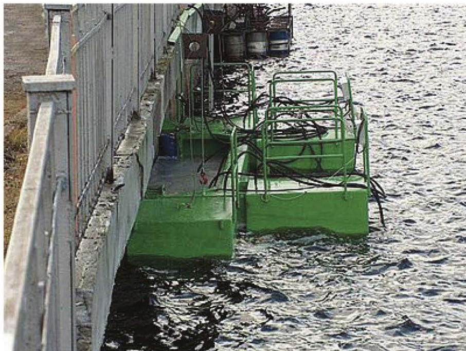
Рисунок 7.4.6 - Металлическая кессонная камера для ремонта структурно поврежденного бетона в зоне переменного уровня воды.
