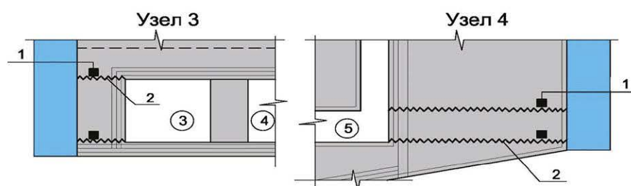
Рисунок 7.1.11 - Типовые узлы гидроизоляции в потернах, цементационных галереях и соединительных коридорах (узлы 3 и 4 на рис. 7.1.10): 1 – гидроизоляционный жгут «Пенебар» и «Скоба крепёжная металлическая»; 2 – шов бетонирования; 3 – цементационная галерея; 4 – дренажная галерея (потерна); 5 – соединительный коридор.
