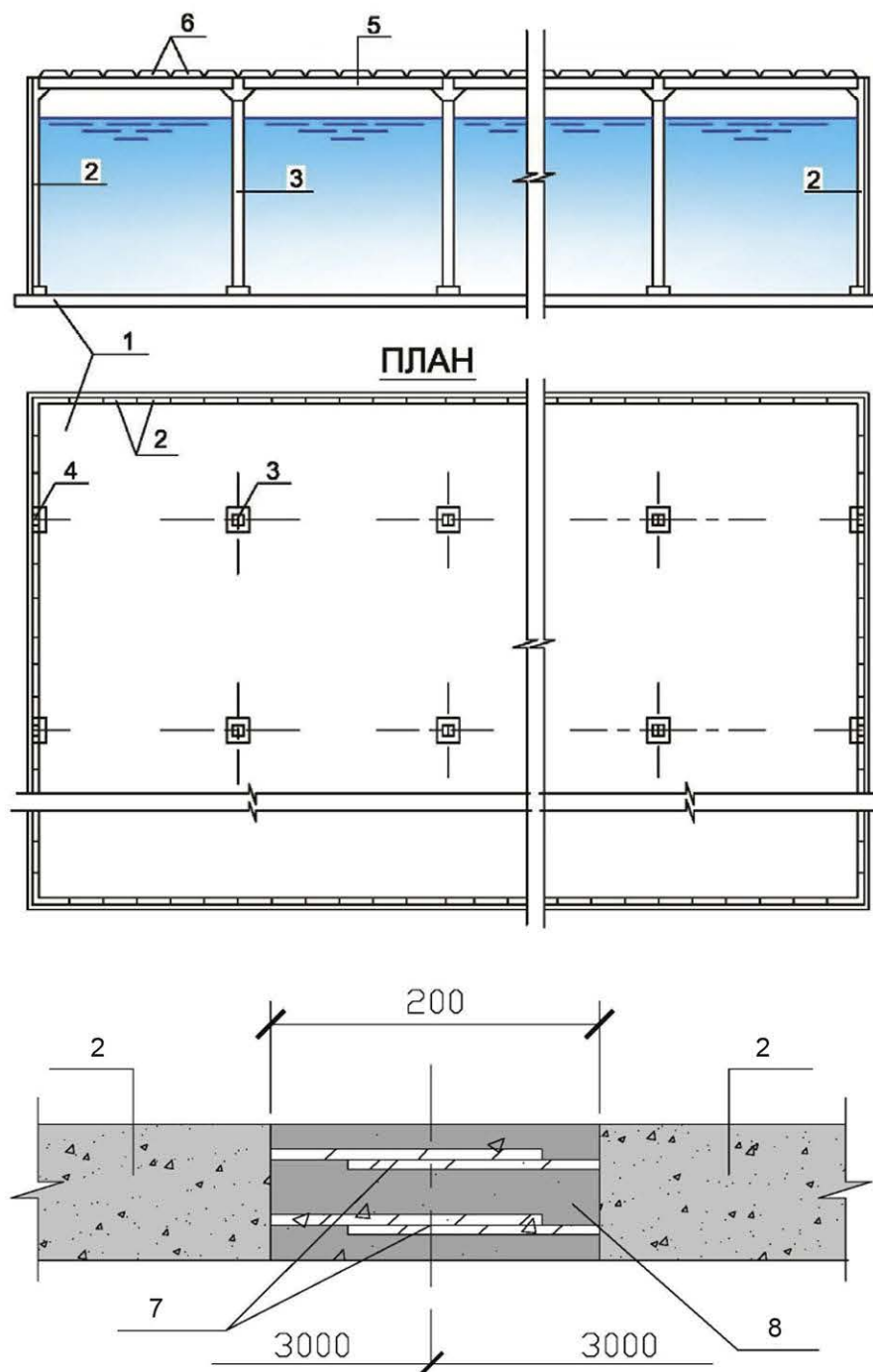
Рисунок 6.4.2 - Схема прямоугольного резервуара из сборных железобетонных панелей:
