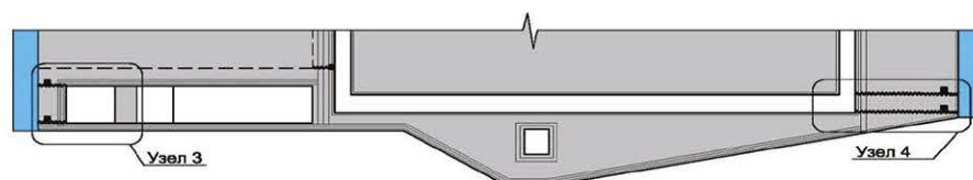
Рисунок 7.1.10 - Схема расположения швов бетонирования и монтажа гидроизоляционного жгута «Пенебар» и «Скобы крепёжной металлической» в местах сопряжения стен и перекрытий в потернах, смотровых шахтах и соединительных коридорах здания ГЭС (фрагмент 2 на рис. 6.1.1).
