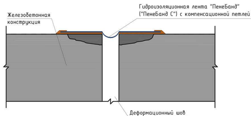
Рисунок 7.3.13 - Монтаж гидроизоляционной ленты «ПенеБанд» («ПенеБанд С»).
