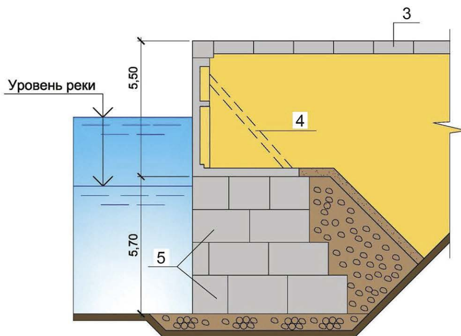
Рисунок 6.5.2 - Конструкция причального сооружения из массивной кладки с надстройкой:
