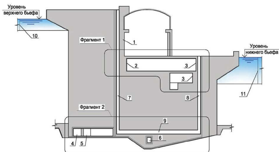
Рисунок 6.1.1 - Руслонное здание ГЭС:
