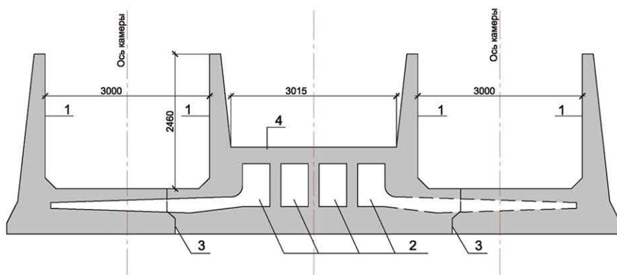
Рисунок 6.3 - Двухниточный судоходный шлюз:
