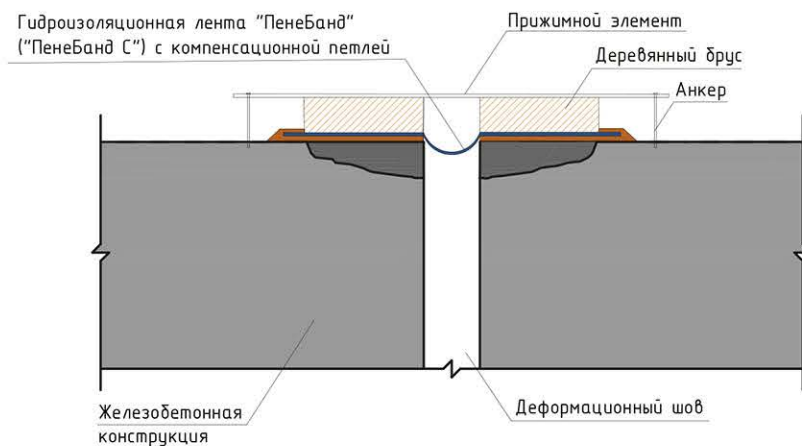
Рисунок 7.3.14 - Прижим гидроизоляционной ленты.
